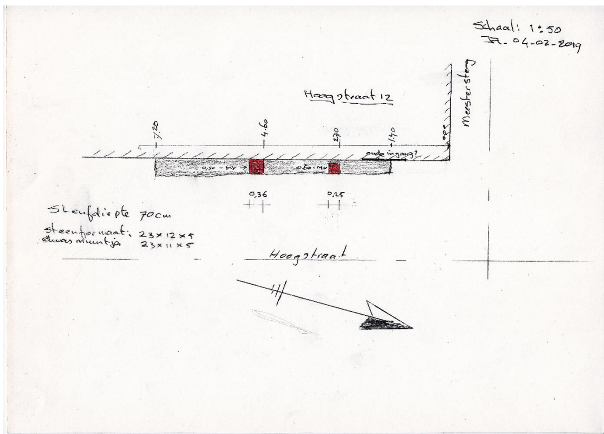
Situatieschets, schaal 1:50
