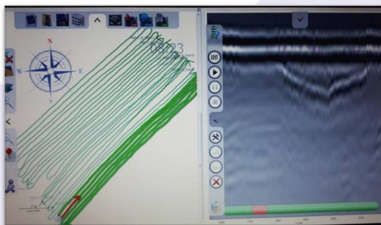
Radarbeelden van de schans, links de gelopen route. Rechts een beeld van de grondradar.
